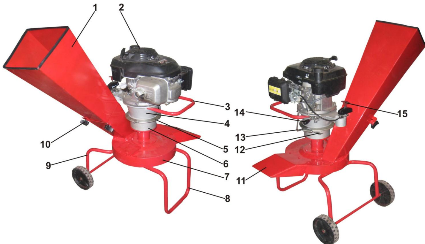
Рис. 1. Измельчитель ИМ-1.
